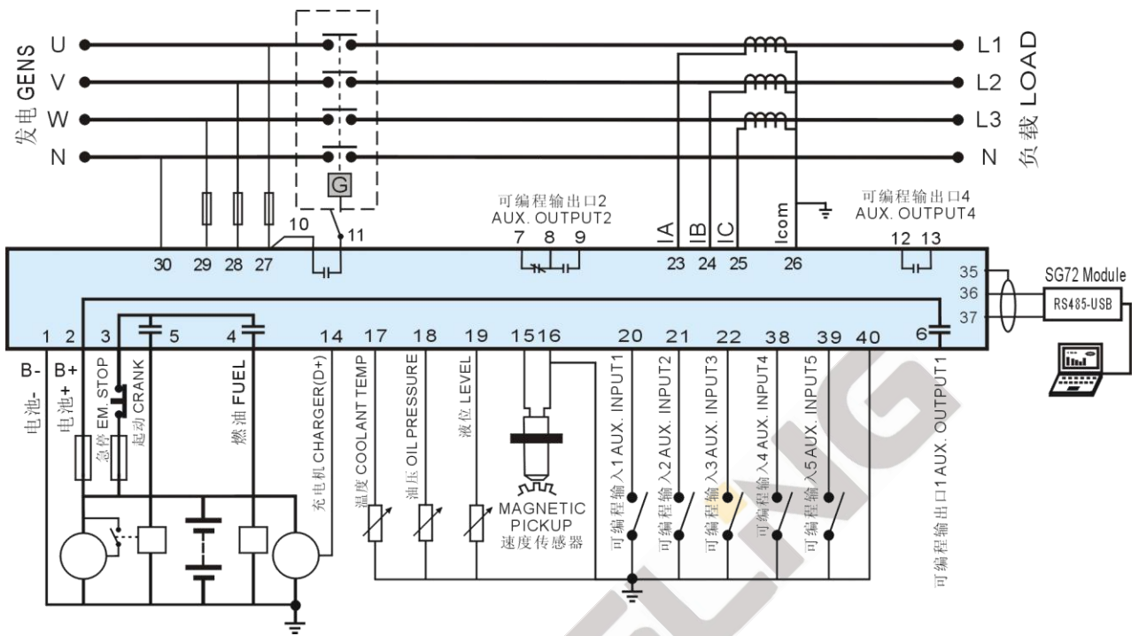
CLE6110UNC 典型应用图
