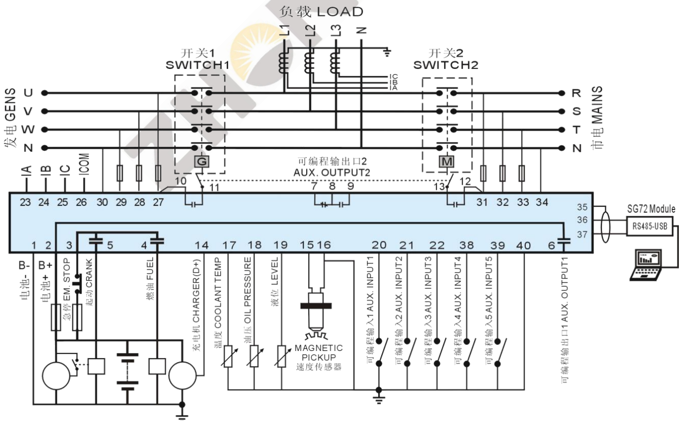
CLE6210UNC 典型应用图
